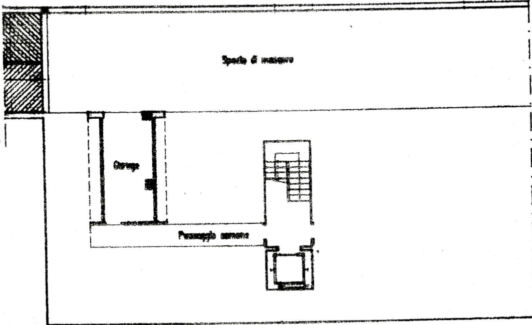
PIANO 1° SOTTOSTRADA h= 2.50 mt
